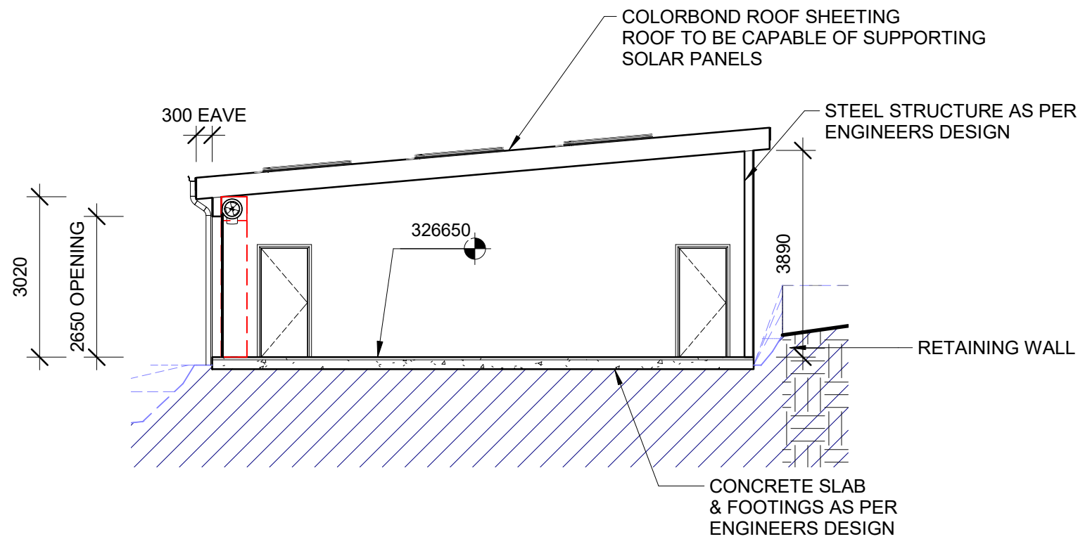
1 Section 5 1 : 100
